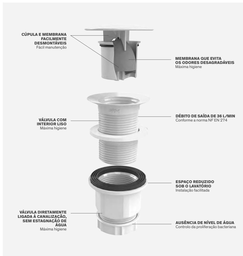
Corte 3D_621W: válvula sem água
